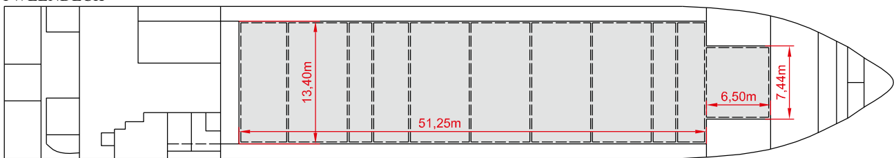
TWEENDECK
